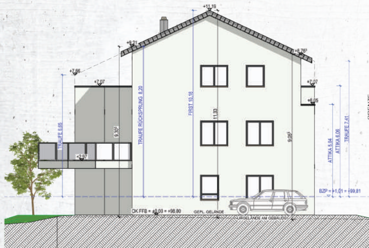
ANSICHT OST
