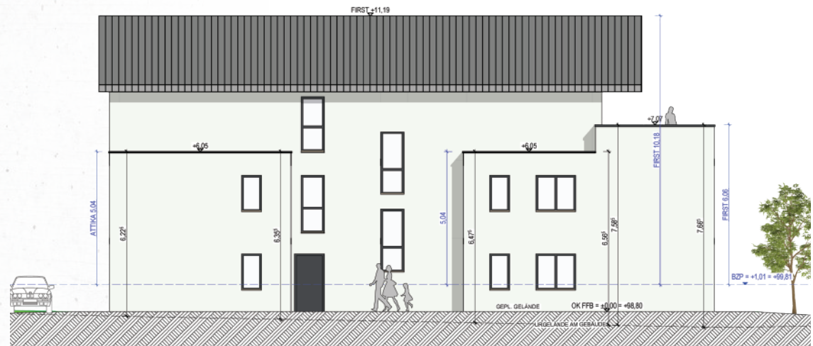
ANSICHT NORD
